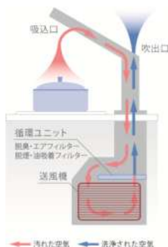
循環式レンジフード 概念図
