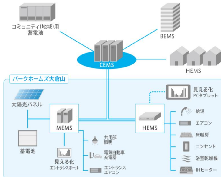
CEMS 概念図
